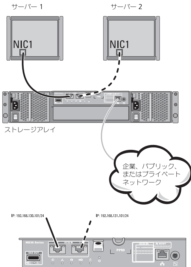
図 2-1. 単一のコントローラに接続された 2 台のホスト
