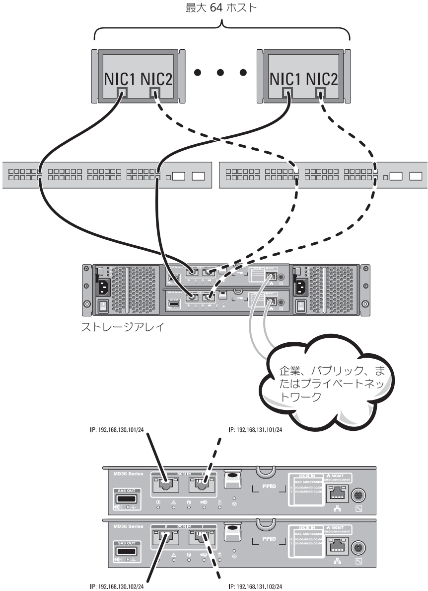
図 2-7. 2つのコントローラに接続された 64 台のサーバー
