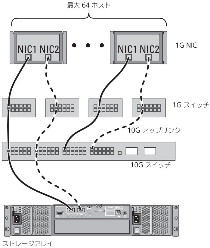
図 2-8. 1つのコントローラに接続された64台のサーバー
