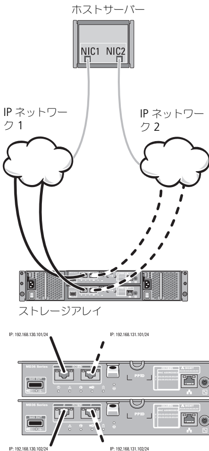
図 C-1. イニシエータの構成
