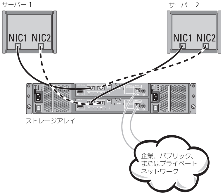
図 2-4. 2つのコントローラに接続された2台のホスト
