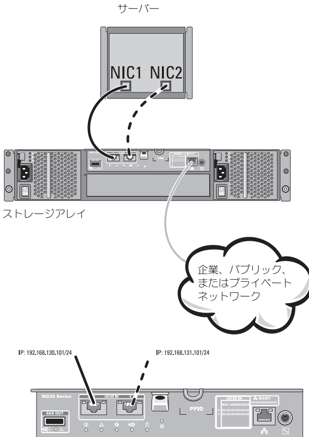
図 2-2. 1 つのコントローラアレイに接続された 1 つのホスト
