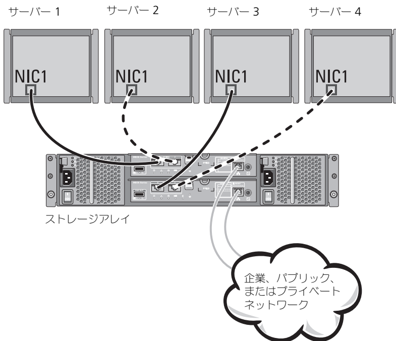
図 2-3. デュアルコントローラ構成の 4 台のホスト
