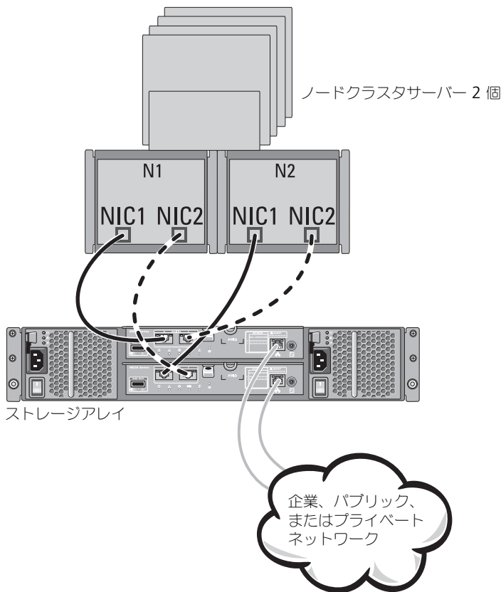
図 2-5. デュアルコントローラ構成で 2 台のホストを接続
