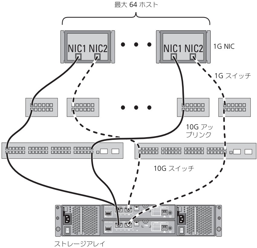
図 2-9. 2つのコントローラに接続された 64 台のサーバー
