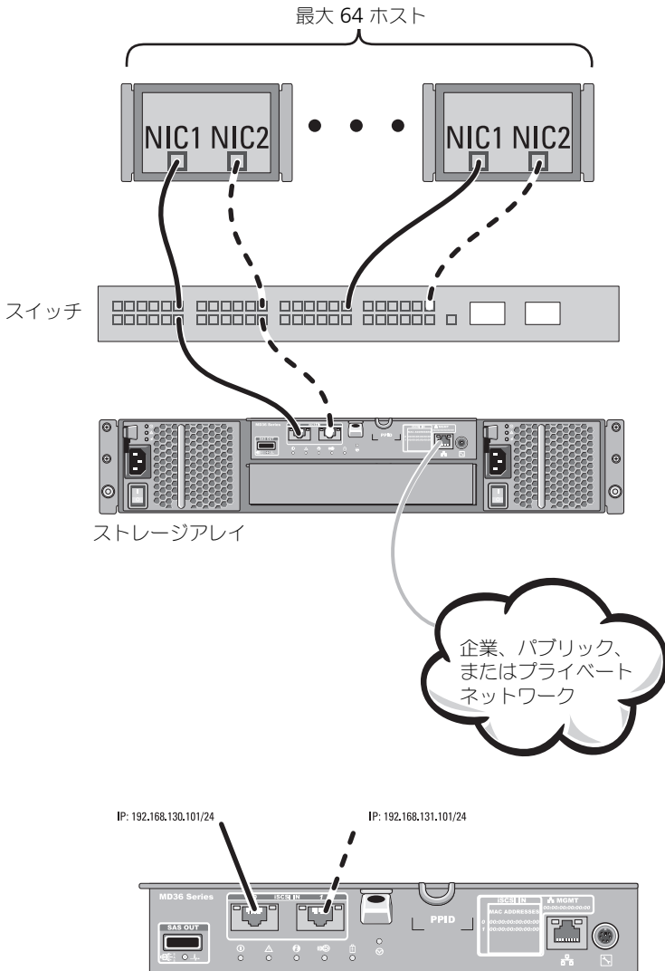
図 2-6. 1つのコントローラに接続された64台のサーバー
